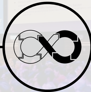
DevOps
